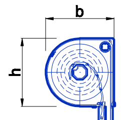
GK-R z moskitierą
